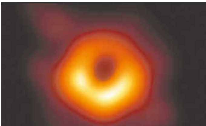
Schwarzen Loch in der Galaxie Messier 87. Foto: Event Horizon Telescope, https://commons.wikimedia.org/wiki/File:Black_hole_-_Messier_87_crop_max_res.jpg
