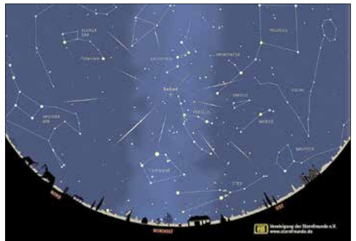
Fluchtpunkt der Perseiden im namensgebenden Sternbild Perseus. Grafik: Vereinigung der Sternfreunde (VdS)
