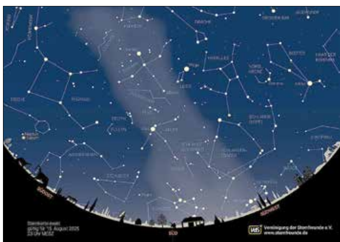
Der Nachthimmel am 15. August um 23 Uhr. Grafik: Vereinigung der Sternfreunde (VdS)
