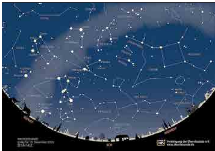
Sternkarte für den 15. Dezember, 22 Uhr. Grafik: Vereinigung der Sternfreunde (VdS)
