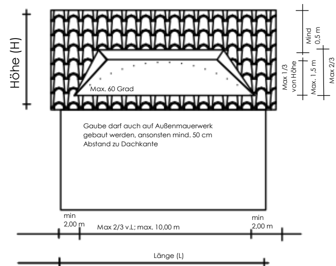
Schleppgauben
