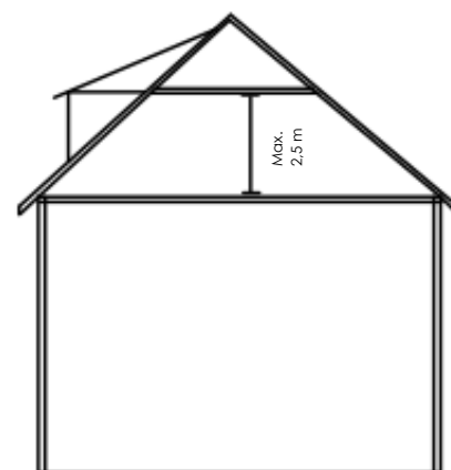
Schleppgauben
